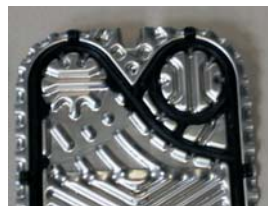
Placa última con junta
